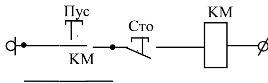
Рисунок. Релейно-контактная схема кнопочной станции.
