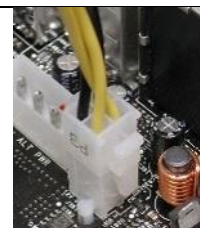
Разъем питания ATX_12V: подключается к разъему ATX_12V на системной плате
