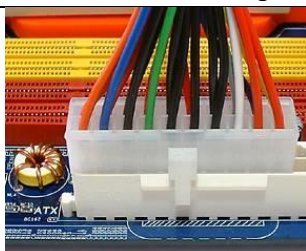
Разъем питания ATX: подключается к разъему ATX на системной плате
