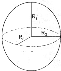
Рис. 1. Форма и размеры Земли
